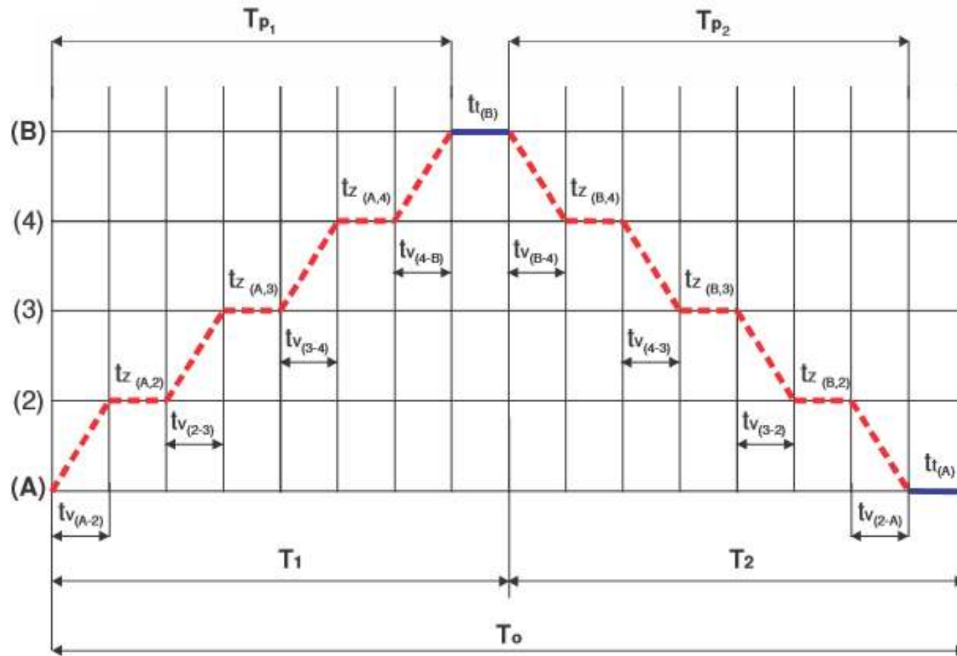
Dijagram PUT-VRIJEME u toku jednog obrta vozila
